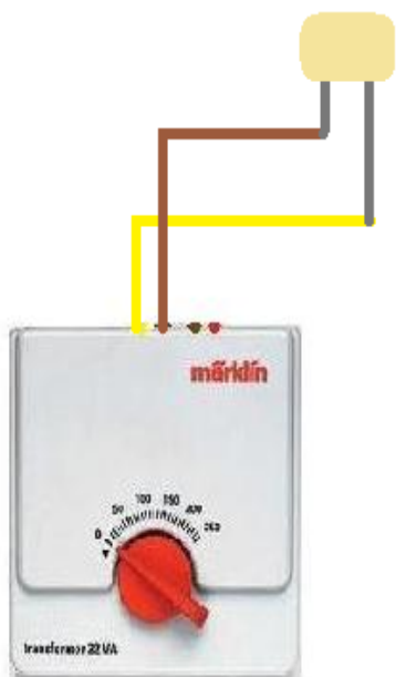
Märklin transformer 6646
